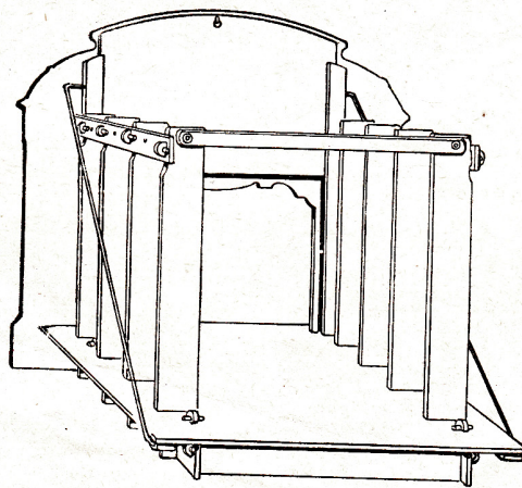
FIG. 2. — Assemblage complet des diverses pièces de charpente de Mon Théâtre.
