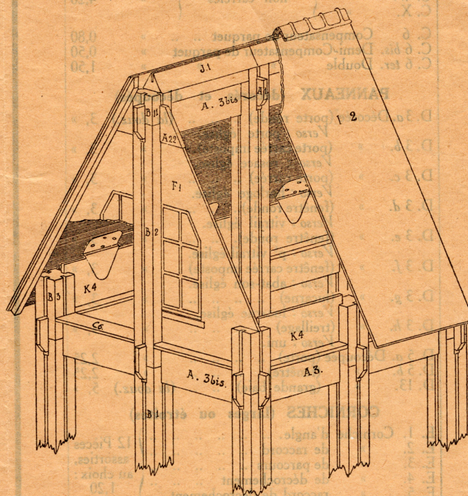
(Fig. 2). Toiture fixée sur la Galerie (K. 4), à l'aide de son crochet métallique.
