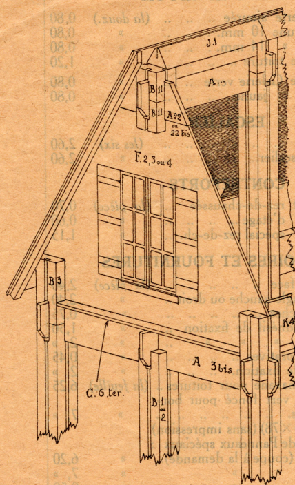
(Fig. 1). Utilisation du double Compensateur de parquet (C. 6 ter) et du Faîtage intérieur (J. 1).
